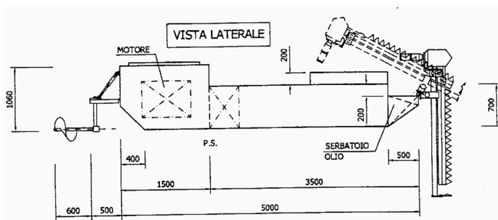
Esempio: Monoelica 5000/1600 ER.EP.SM.T.
